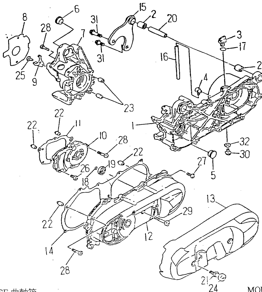
FIG.07 CRANKCASE 曲軸箱
