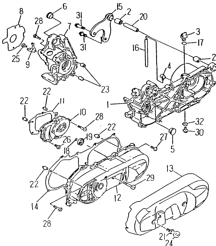
FIG.07 CRANKCASE 曲軸箱
