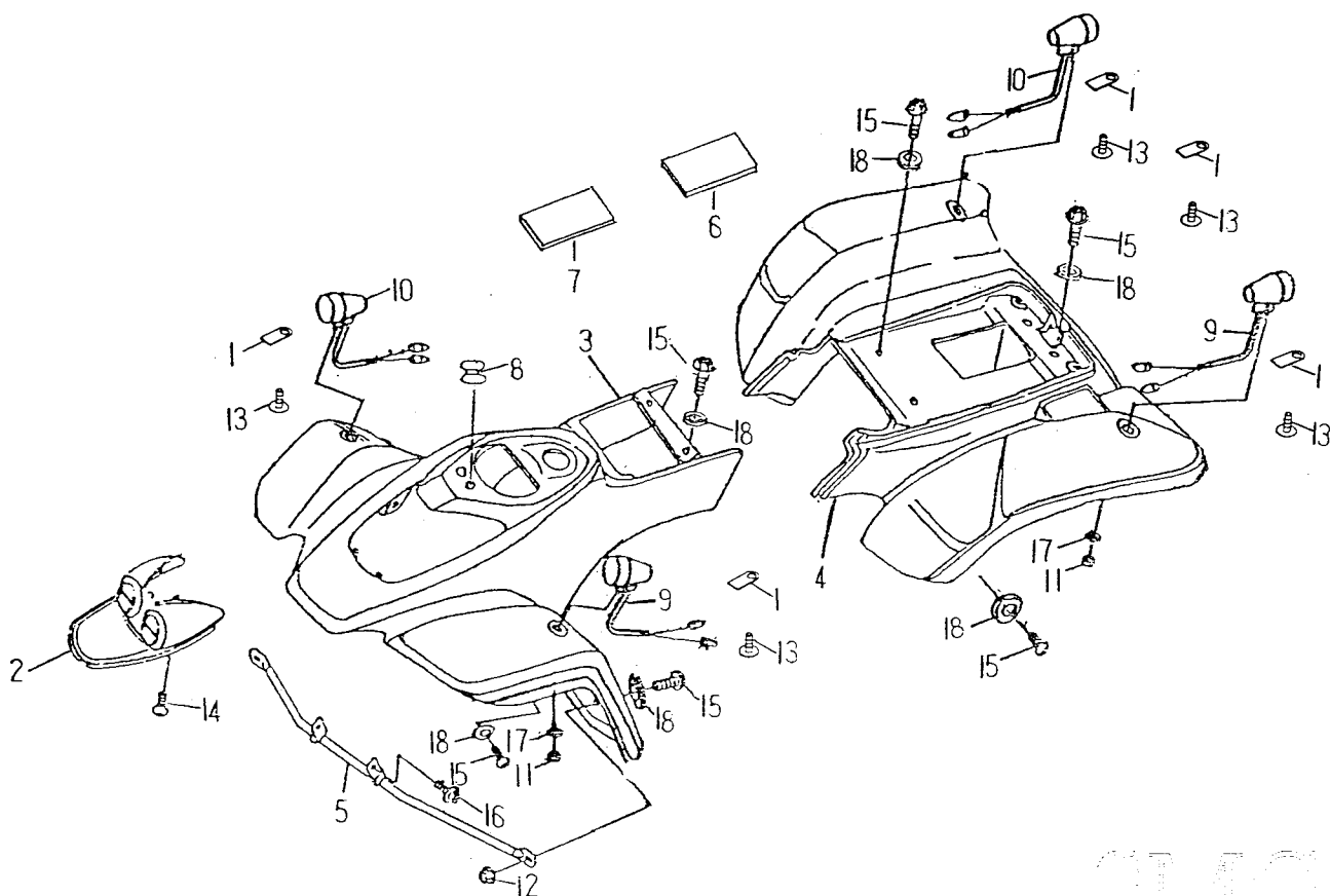
FIG.20 FRONT FENDER 前土除
