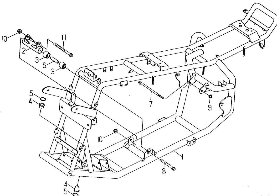
FIG.16 FRAME 車架
