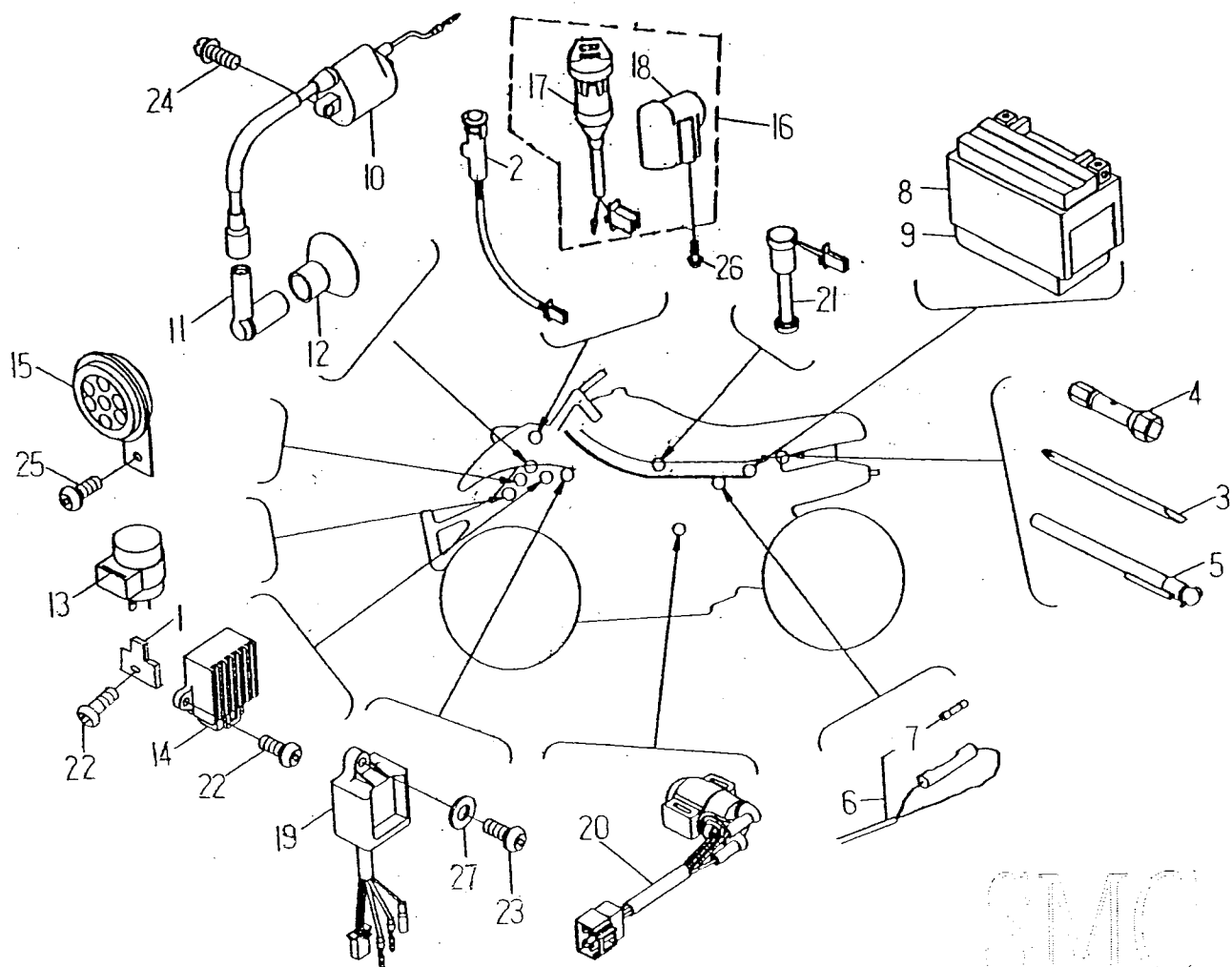
FIG.29 WIRE HARNESS 主電路配線
