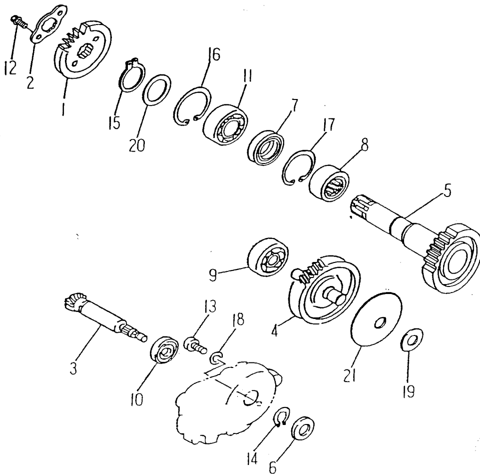
FIG.10 TRANSMISSION 傳動機構
